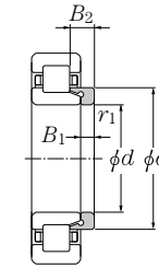
NH=NJ+HJ
